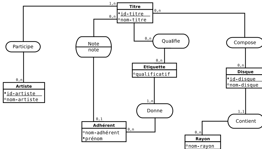
FIGURE 2 – Modèle conceptuel de données
